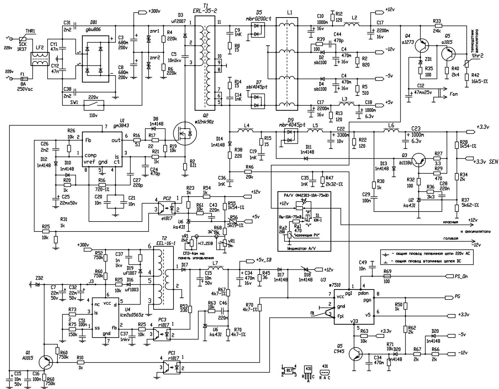
Зарядное устройство из блока питания "Power Man IP-P350AJ". Схема электрическая принципиальная.
